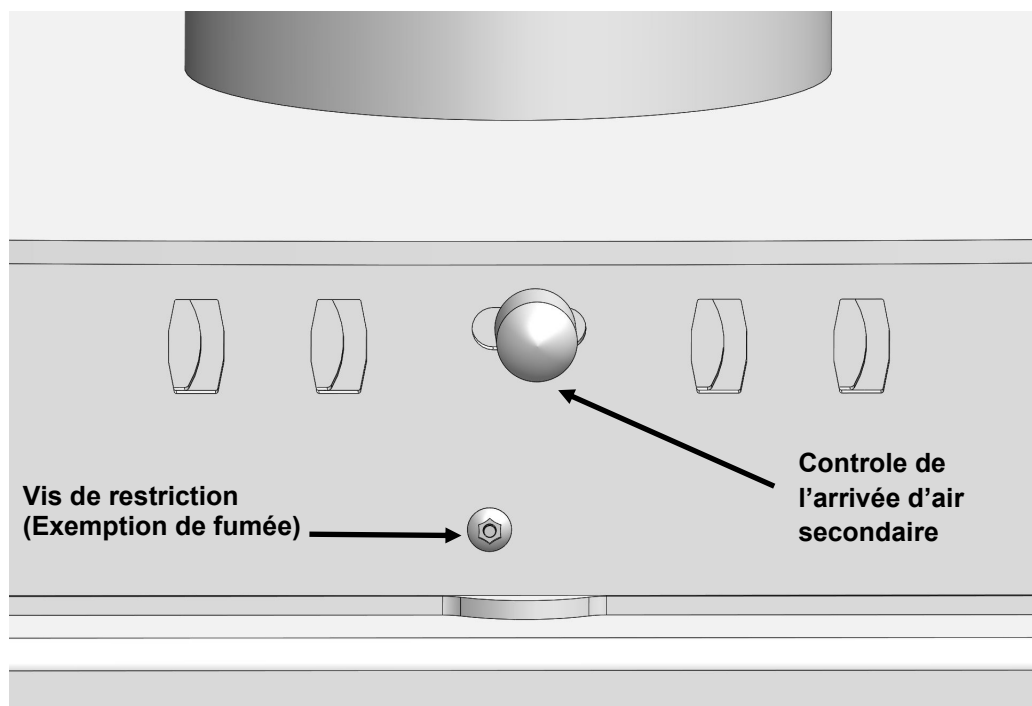
Fig. 5. Vis de restriction anti-fumée installée
